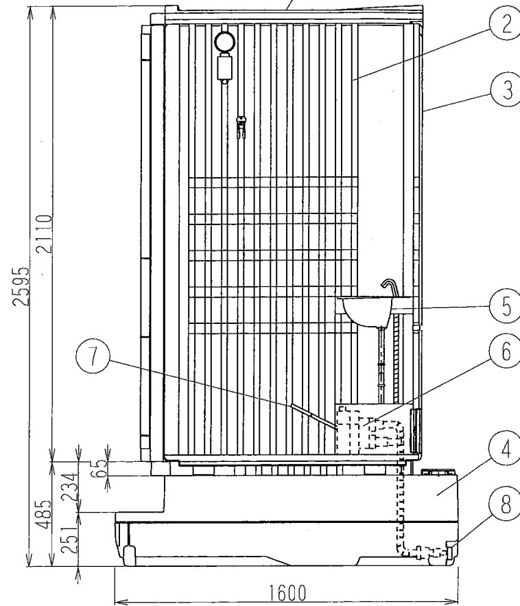
側面図
