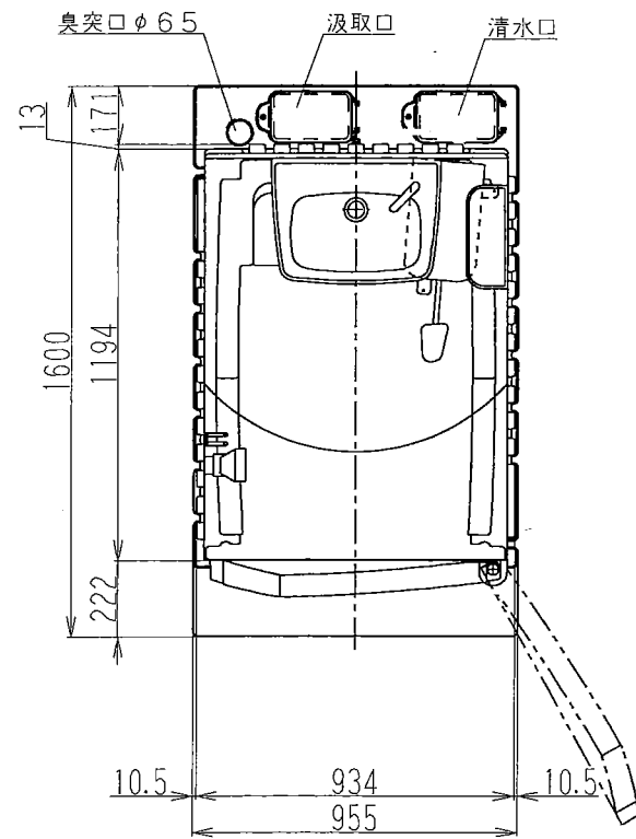
平面図
