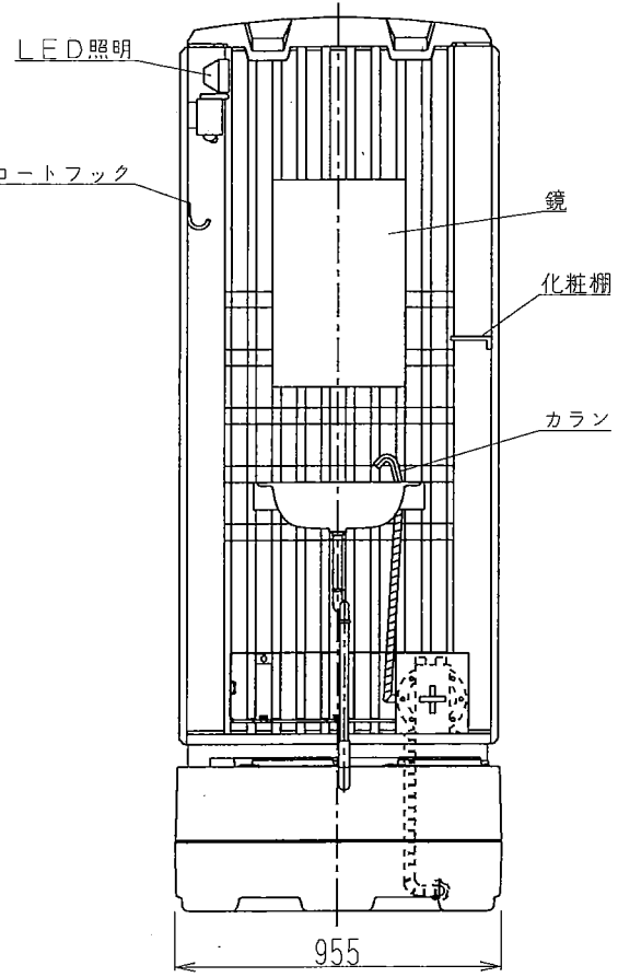
正面図
