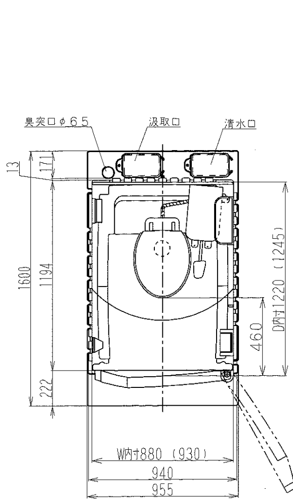
平面図
