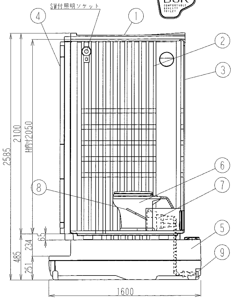
側面図
