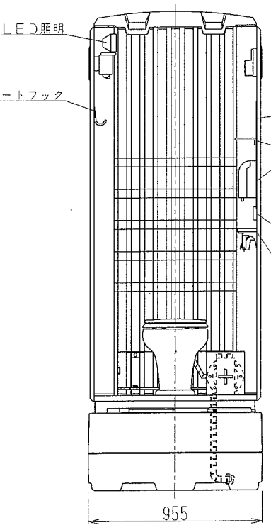
正面図
