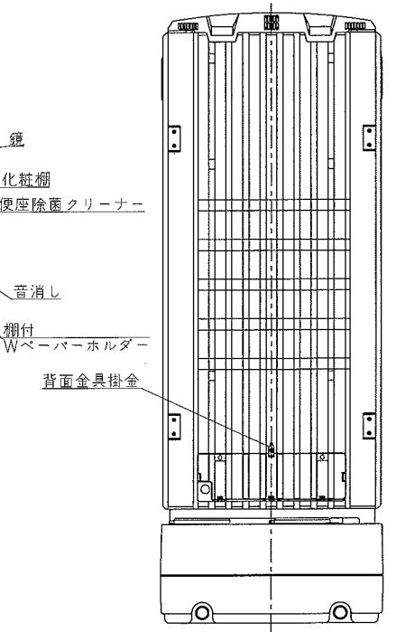
背面図
