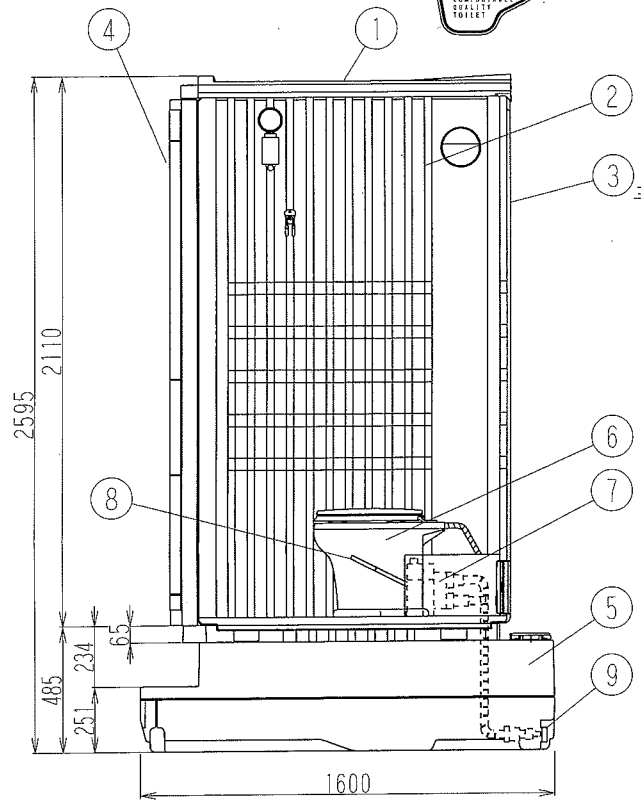
側面図
